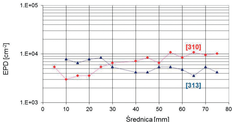
Rys. 3. Rozkład gęstości dyslokacji w kryształcie o średnicy 3" na płaszczyźnie (310) wzdłuż kierunków [310] i [313].
