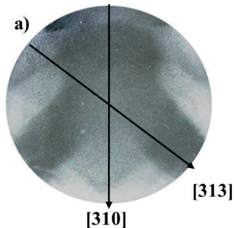
Rys. 2. Makroskopowy obraz struktury dyslokacyjnej monokryształu SI GaAs o średnicy 2" i orientacji [310]; jasne pola – obszary o wyższej gęstości dyslokacji.
