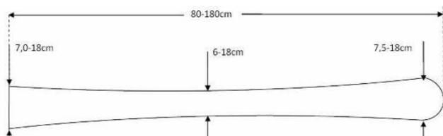
Rys. 1. Geometria narty (widok z góry) [5]
