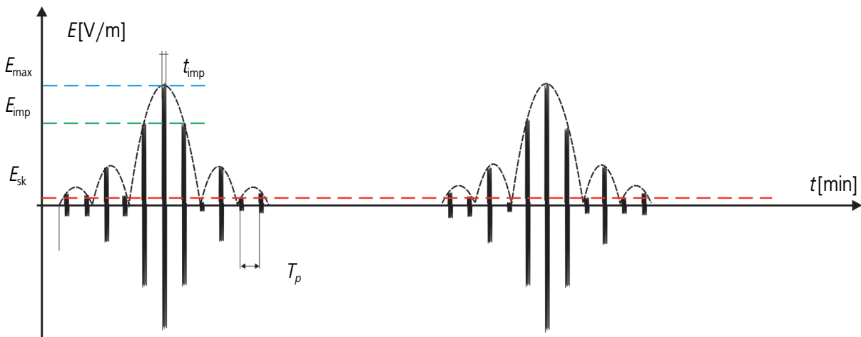
Rycina 6. Natężenie pola elektrycznego w punkcie pomiarowym w funkcji czasu podczas pomiarów radaru (odległościomierza), gdzie E_{max} – wartość szczytowa natężenia pola elektrycznego, E_{imp} – maksymalna wartość skuteczna natężenia pola elektrycznego uśredniona w czasie trwania impulsu, E_{sk} – wartość skuteczna w okresie realizacji pomiarów, t_{imp} – czas trwania impulsu, T_p – okres repetycji impulsów Figure 6. Electric field strength at the measuring point as a function of time during radar (surveillance radar) measurements, where E_{max} – the peak value of the electric field strength, E_{imp} – the maximum rms value of the electric field strength, averaged during the pulse duration, E_{sk} – rms value during the measurement period, t_{imp} – pulse duration, T_p – pulse repetition period
