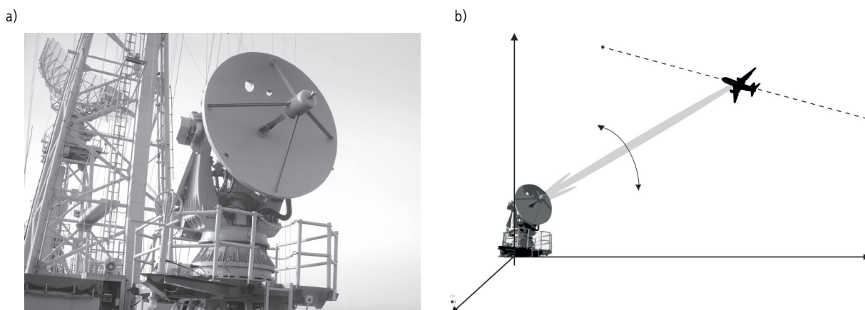
Rycina 5. Radar kierowania ogniem: a) widok ogólny, b) charakterystyka wiązki i zasada śledzenia obiektu Figure 5. Fire control radar: (a) general view, (b) beam characteristics and object tracking principle
