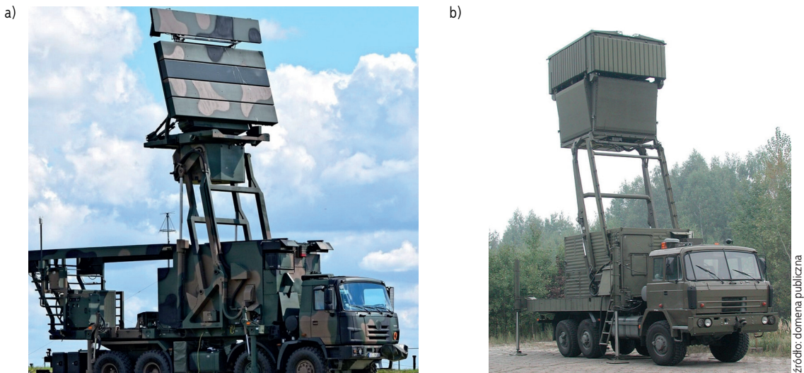
Rycina 3. Radary typu trójwspółrzędnego: a) widok radaru quasi-trójwspółrzędnego, b) widok rzeczywistego radaru trójwspółrzędnego Figure 3. 3D radars: a) view of a quasi-3D radar, b) view of an actual 3D radar
