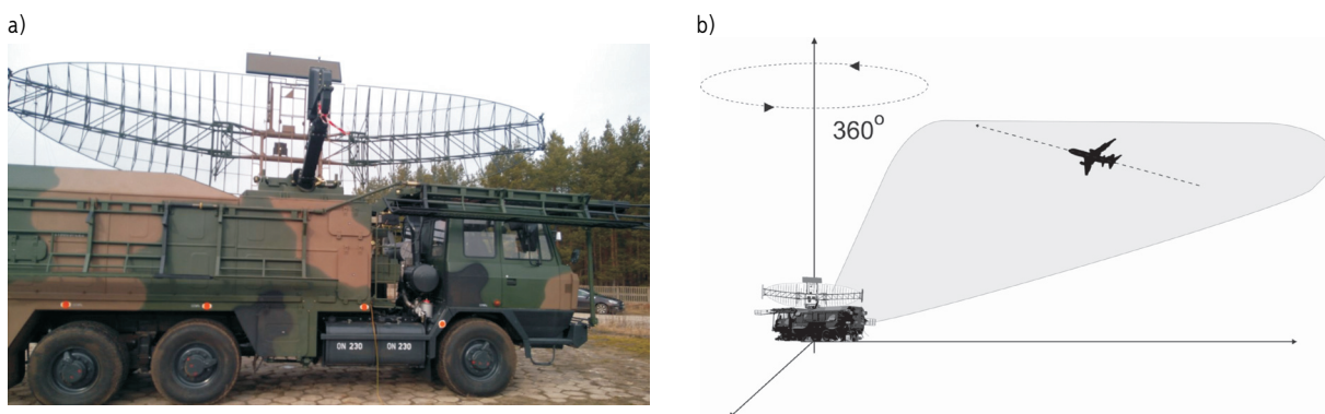
Rycina 1. Radar typu odległościomierz: a) widok ogólny, b) charakterystyka promieniowania i specyfika pracy dookólnej Figure 1. Surveillance type radar: (a) general view, (b) radiation characteristics and omnidirectional operation specification
