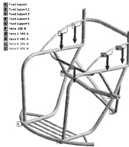
Rys. 9. Model z zaznaczonymi powierzchniami przyłożenia sił
