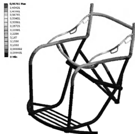
Rys. 10. Model z nałożoną mapą naprężeń
