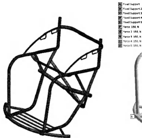
Rys. 8. Model z nałożoną siatką elementów skończonych
