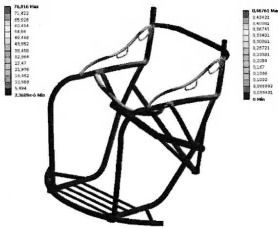
Rys. 10. Model z nałożoną mapą naprężeń
