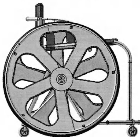
Rys. 6. Wirtualny model wózka inwalidzkiego sportowego – widok z prawej
