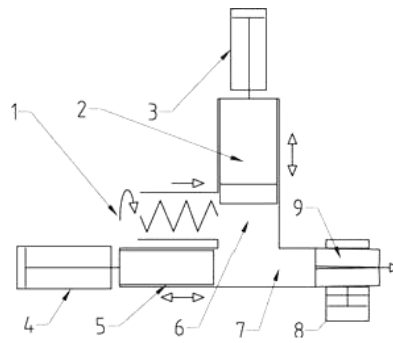
Fig. 1. Scheme of a hydraulic briquette press
