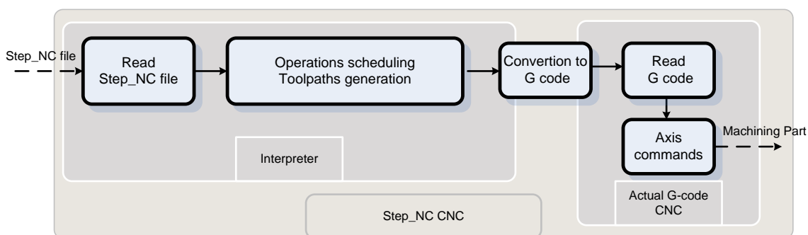
Fig. 7. Interpreted Step_NC programming
