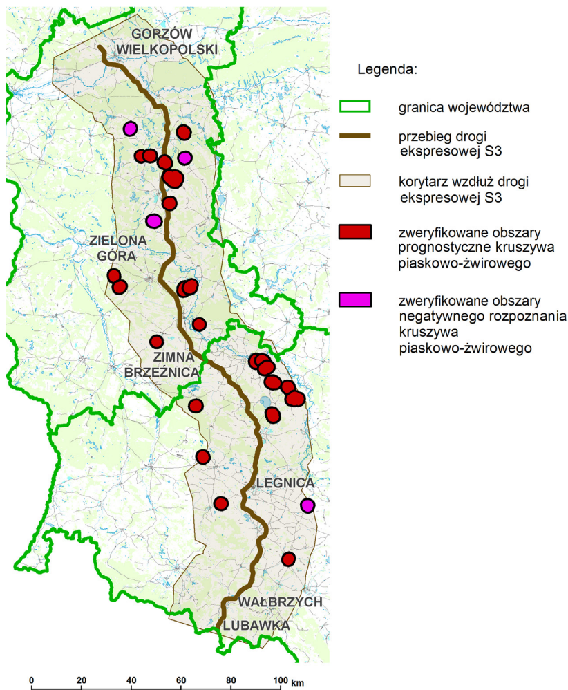
Rys. 3. Mapa rozmieszczenia zweryfikowanych obszarów prognostycznych i negatywnych kruszyw piaskowo-żwirowych wzdłuż drogi ekspresowej S3 na odcinku Gorzów Wielkopolski–Lubawka
