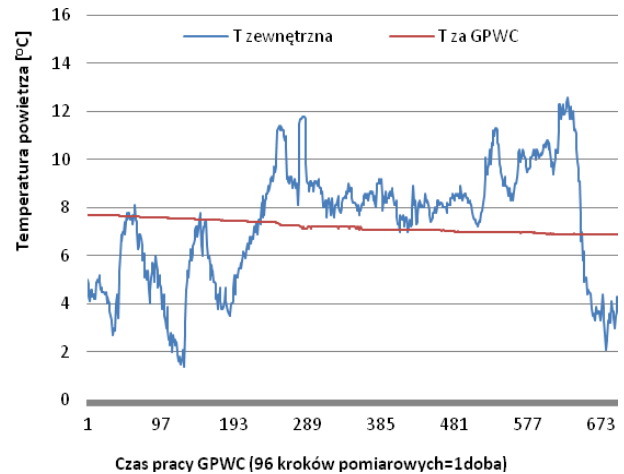
Rys. 8. Wykres temperatury powietrza zewnętrznego i po przejściu przez GWPC w grudniu 2015 roku
