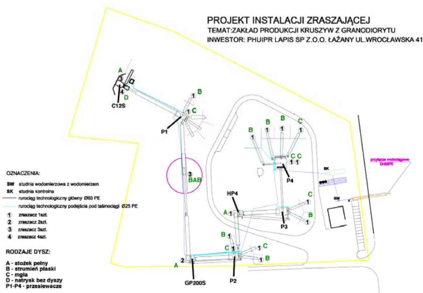
Rys.1. Plan rozmieszczenia natrysków wodnych w instalacji zraszającej zakładu przeróbczego Kopalni Granodiorytu Łażany (autor: Tomasz Jaworski)
