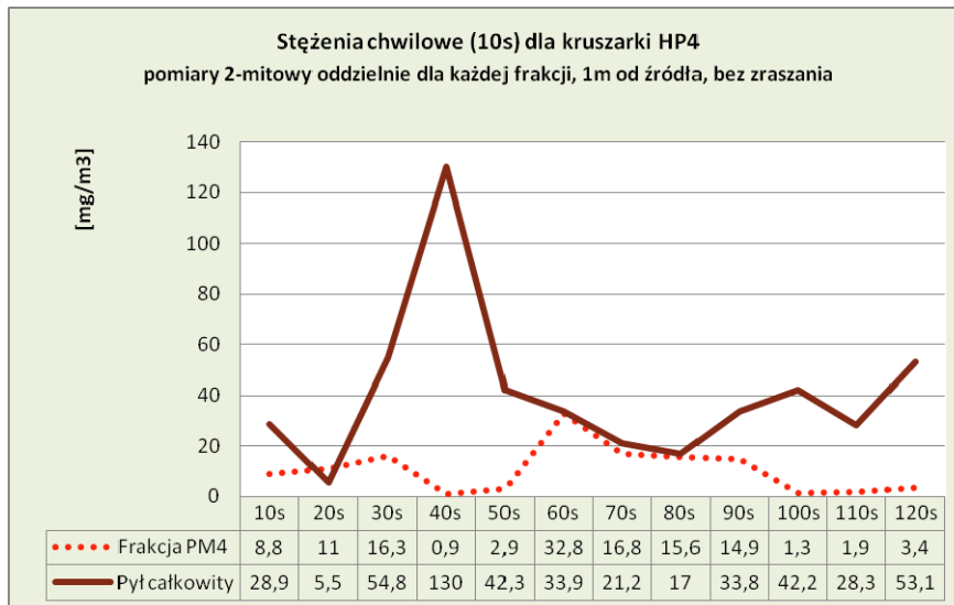
Rys. 7. Zmiana stężenia pyłu w czasie 2- minut dla kruszarki HP4, pomiar 1 m od wysypu z kruszarki na przenośnik Fig. 7. Change in dust concentration during two minutes for crushers HP4, measured 1m from the crusher discharge conveyor
