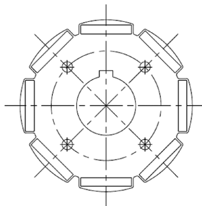
Rys. 2. Kształt blachy wirnika
