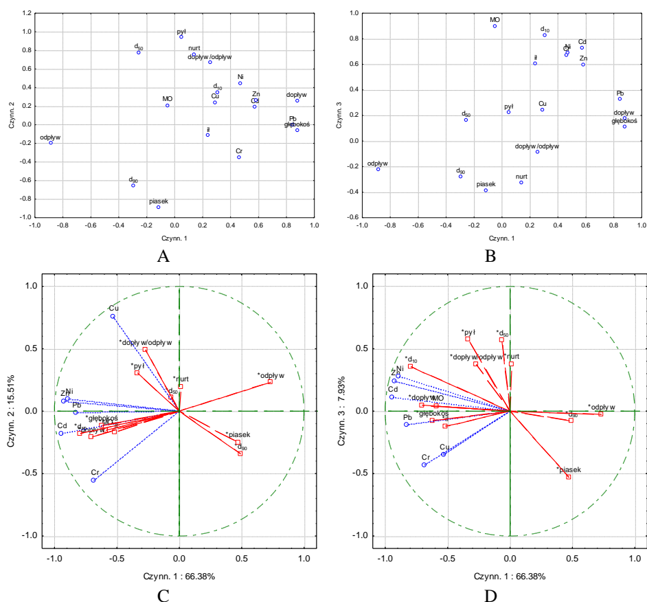
Rys. 5. Analiza składowych głównych stężeń metali ciężkich w osadach dennych wstępnej części zbiornika Stare Miasto
