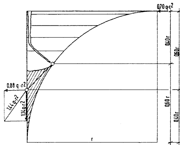
Rys. 7. Schemat zarysowania sklepienia wg Piepera
