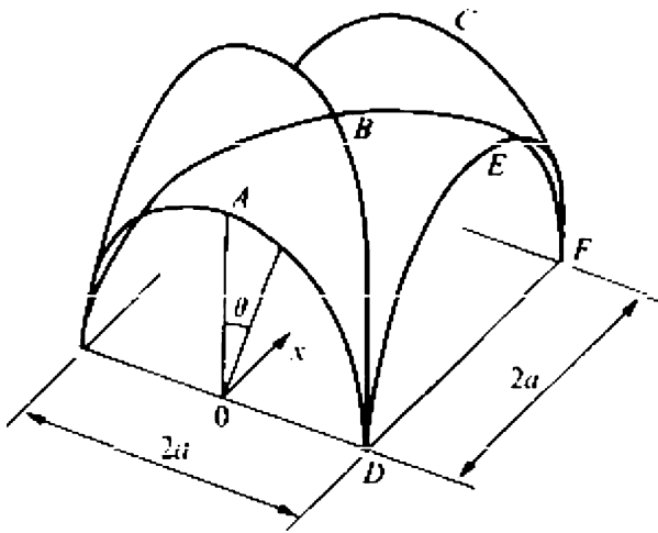
Rys. 9. Model sklepienia żeberowego
