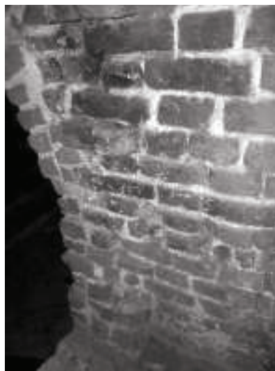
Ryc. 15. Okopczenia widoczne na powierzchni licowej zachodniej ściany komory wewnętrznej pieca. Fot. A.Bojęś-Białasik, 2009 Fig. 15. Soot black visible on the face of the west wall of the internal stove chamber. Photo by A. Bojęś-Białasik, 2009
