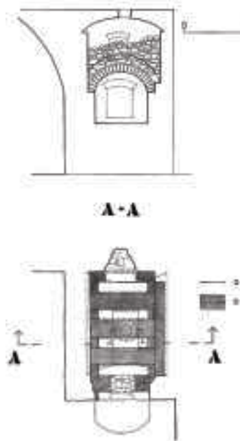
Ryc. 18. Rekonstrukcja pieca typu hypocaustum we wschodnim skrzydle klasztoru augustianów w Krakowie. Oprac. A. Bojęś-Białasik Fig. 18. Reconstruction of the hypocaustum type stove in the east wing of the Augustinian monastery in Krakow. Made by A. Bojęś-Białasik
