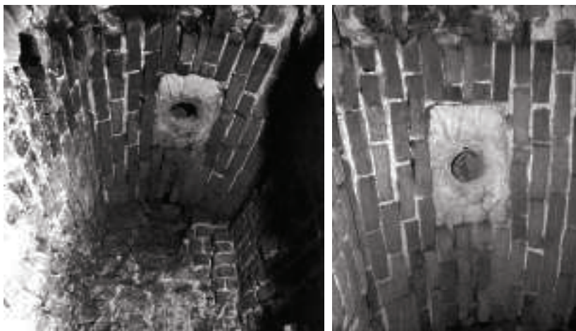
Ryc. 14. Klasztor augustianów w Krakowie, piec w piwnicy skrzydła wschodniego; widoczny cios wapienny z otworem wlotowym gorącego powietrza, umieszczony w podniebieniu sklepienia pieca. Fot. archiwalna T. Szklarczyk 1989, fot. stanu obecnego A. Bojęś-Białasik, 2009 Fig. 14. Augustinian monastery in Krakow, the stove in the east wing cellar; a limestone block with an inlet for hot air is visible, located in the soffit of the stove vault. Photo: archive, by T. Szklarczyk 1989, photo of the present state by A. Bojęś-Białasik, 2009
