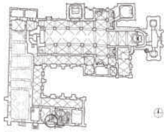
Ryc. 2. Klasztor cystersów w Jędrzejowie, stan dzisiejszy przyziemia z naniesionym rzutem piwnic pod dawnym refektarzem, na czerwono oznaczono lokalizację urządzenia piecowego. Oprac. B. Kwiatkowska-Kopka Fig. 2. The Cistercian monastery in Jędrzejów, present state of ground level with the marked projection of cellars under the old refectory, location of the heating device was marked in red. Made by B. Kwiatkowska-Kopka
