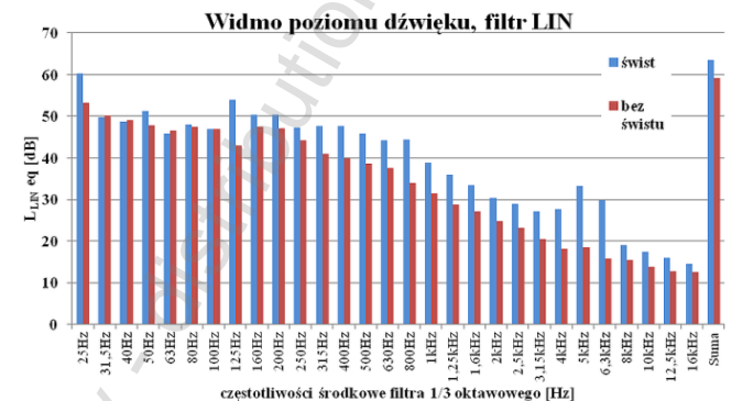
Rys. 3. Porównanie poziomów równoważnych dźwięku dla pomiaru, w którym występowały słyszalne świsty i pomiaru bez świstów, 100 m od turbiny, 1,5 m n.p.t., czas pomiaru 1 min
