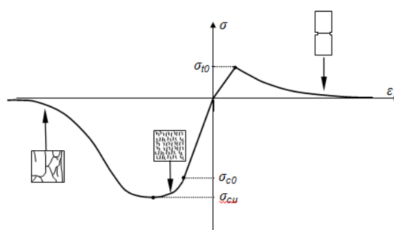
Rys. 1. Wykres naprężenie - odkształcenie w próbach jednoosiowego ściskania i rozciągania wraz ze wskazaniem miejsc powstania pęknięć dla typowego materiału quasi-kruchego [Małyszko & Orłowicz 2000]
