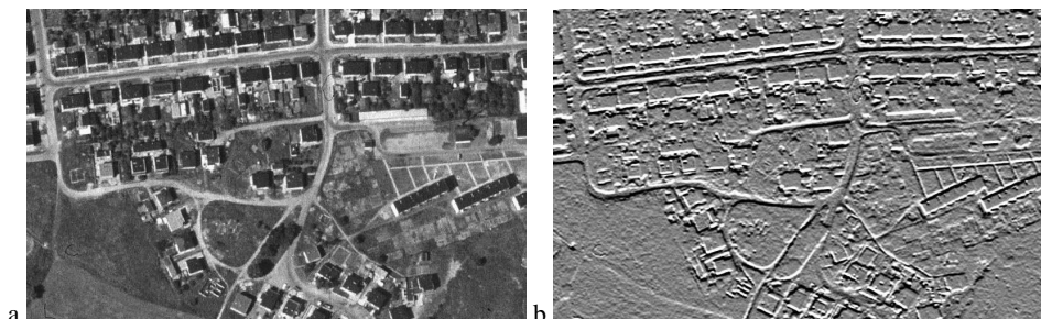
Rys. 1. Sposób wykrywania krawędzi na tonalnym obrazie terenu zabudowanego, przy użyciu operatora Sobela: (a) oryginalny obraz tonalny, (b) uwypuklone krawędzie
