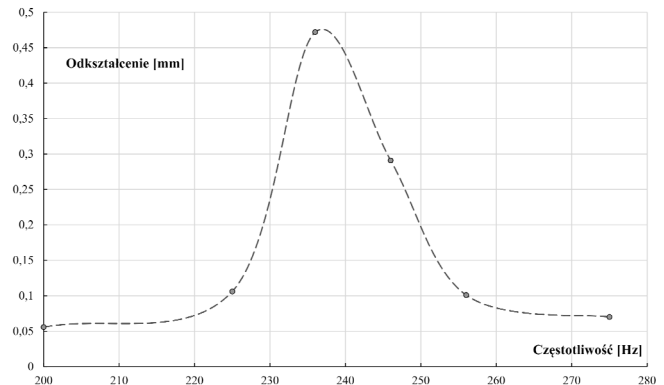
Rys. 3. Odkształcenia maksymalne prototypu I dla częstotliwości rezonansowej
