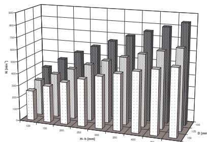
Rys. 5. Optymalne częstotliwości obrotowe
