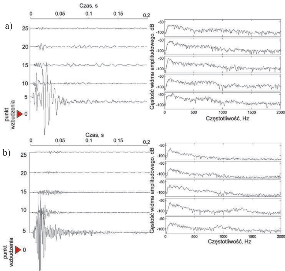
Rys. 2. Sejsmogram (lewa strona) oraz jego widmo amplitudowe (prawa strona) zarejestrowany w wyniku uderzenia młotem w pręt przyłożony do ocisu w wyrobisku dolowym wykonanym w warstwie piaskowca – a i w pokładzie węgla – b
