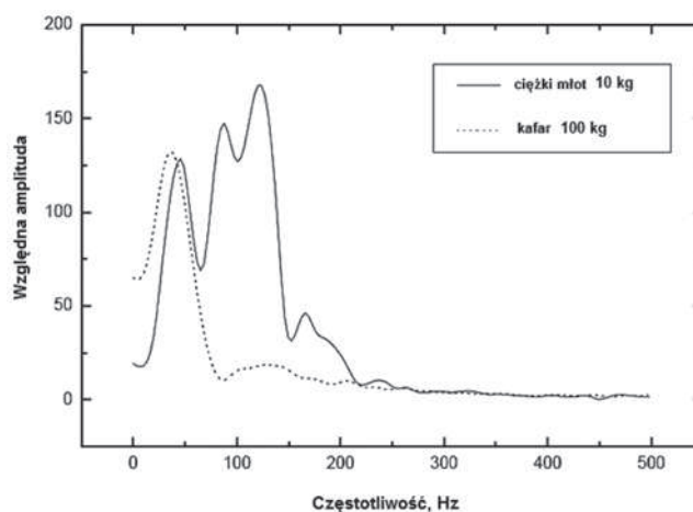
Rys. 6. Porównanie odpowiedzi amplitudowej dla uderzenia młotem o masie 10 kg w metalową płytkę i dla uderzenia kafarem o masie 100 kg bez płytki na podstawie [6]
