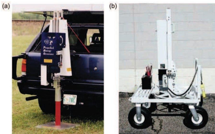
Rys. 5. Przykładowe kafary: Propped Energy Generator produkcji R.T Clark na podstawie [33] – a, ESS100 HM produkcji GISCO na podstawie [31] – b
