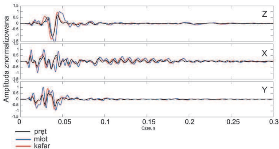
Rys. 8. Porównanie trójskładowej rejestracji fali sejsmicznej wzbudzonej źródłami jak na rysunku 5 w identycznych warunkach pomiarowych, w odległości 4 m od źródła
