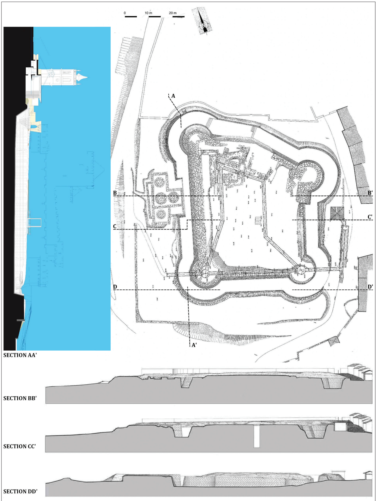
7. Topografia reliktyw zamku, plan i przekroje stanu obecnego na tle projektu urbanistycznego. Oprac. autor 7. Topographical survey of the remains of the castle, plan and sections of the present state, with the urban design of the site. Prepared by the author
