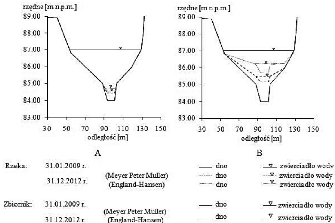
Rys. 4. Przekrój poprzeczny 4,810 w warunkach przepływu średniego SSQ = 0,63 m 3 ·s -1 (A) i przepływu maksymalnego WWQ = 6,08 m 3 ·s -1 (B) dla lat 2009–2012 Fig. 4. Cross-section 4,810 for flow 0,63 m 3 ·s -1 (A) and for flow 6,08 m 3 ·s -1 (B) in period 2009–2012
