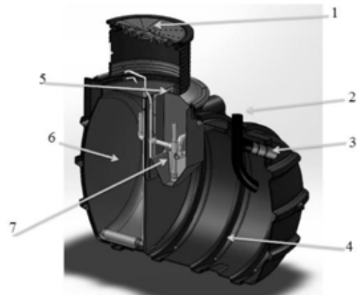
Rys. 2. Budowa biologicznej oczyszczalni ścieków (BioPura) [7]: 1 – pokrywa z tworzywa, 2 – odpowietrzenie, 3 – dopływ ścieku, 4 – osadnik wstępny, 5 – recyrkulacja osadu, 6 – jedna z dwóch stref oczyszczania tlenowego, 7 – osadnik wtórny
