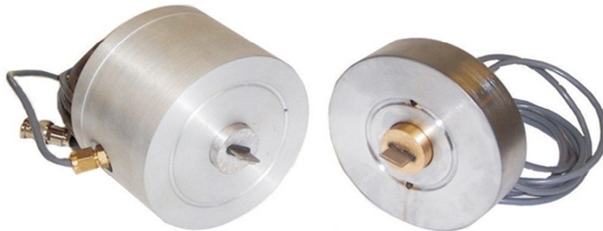
Rys. 2. Cylindry z widocznymi elementami piezoelektrycznymi używane w badaniu propagacji fal w warunkach laboratoryjnych w aparacie trójosiowego ściskania ( http://geotechpedia.com/Equipment/Show/211/Bender-elements ).
