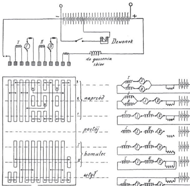
Rys. 2. Schemat walca regulującego
