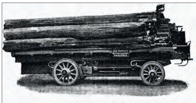
Rys. 11. Ciężarówka „Scheele”
