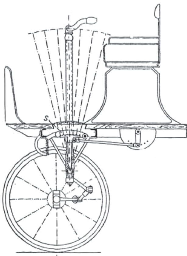
Rys. 4. Układ sterowniczy auta „Victoria”
