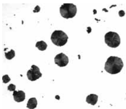
Rys. 10. Grafیت w żeliwie wyjściowym przed obróbką cieplną. Wlewek 75 mm. Pow. 100×, nietraw.
