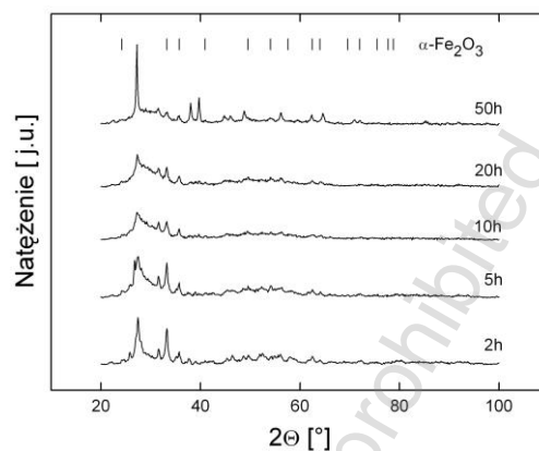
Rys. 2. Zestawienie dyfraktogramów ceramiki (\text{BiFeO}_3)_{0.9}\text{--}(\text{BaTiO}_3)_{0.1} dla próbek mielonych przez 2-50 h. Zaznaczono położenie linii dla \alpha\text{-Fe}_2\text{O}_3
