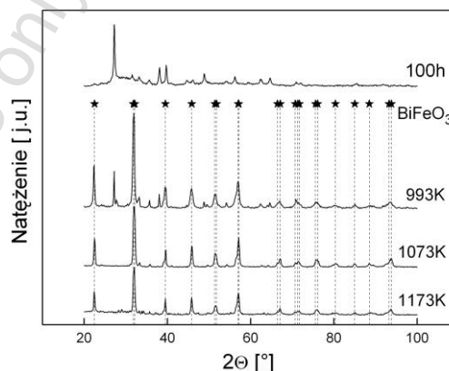
Rys. 3. Zestawienie dyfraktogramów ceramiki (\text{BiFeO}_3)_{0.9}\text{--}(\text{BaTiO}_3)_{0.1} dla próbki mielonej przez 100 h a następnie nagrzewanej do 993 K oraz wygrzewanej w 1073 K i 1173 K. Znakami * zaznaczono położenie linii dla \text{BiFeO}_3 (JCPDS PDF 20-0169)
