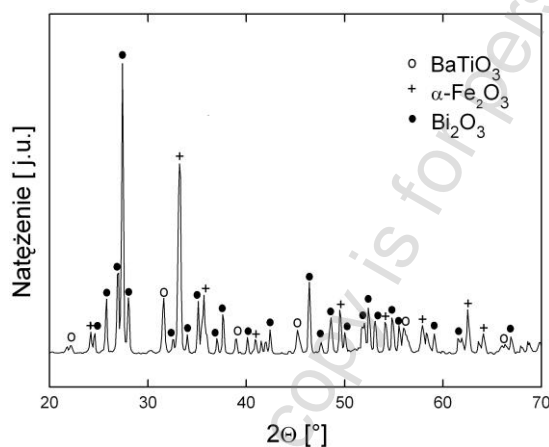
Rys. 1. Dyfraktogram dla mieszaniny wyjściowej składników ceramiki (\text{BiFeO}_3)_{0.9}\text{--}(\text{BaTiO}_3)_{0.1}
