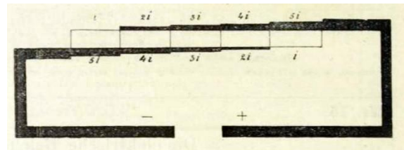
Rys. 4. Sposób dobierania grubości przewodów do poszczególnych lamp w systemie oświetleniowym Gülchera
