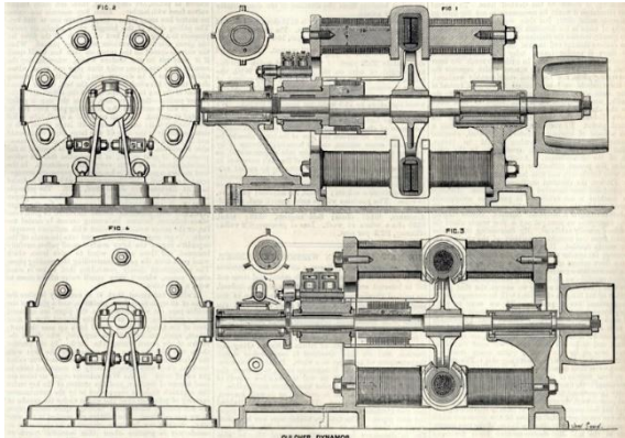
Rys. 2. Rysunki do dynamomaszyny Gülchera
