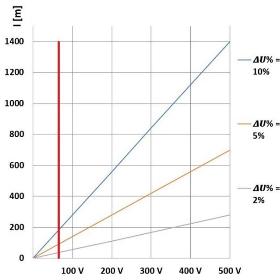
Rys. 7. Wykres zależności l = f(U) , dla s = 2 \text{ A/mm}^2 , czerwoną linią zaznaczono 65 V, napięcie systemu Gülchera
