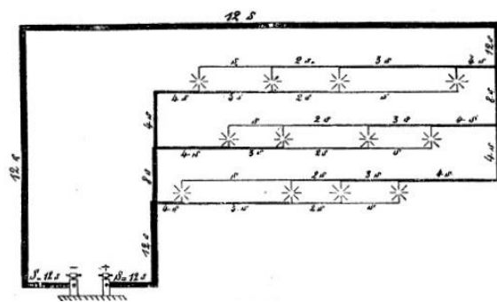
Rys. 3. Schemat połączenia równoległego lamp łukowych w systemie Gülchera
