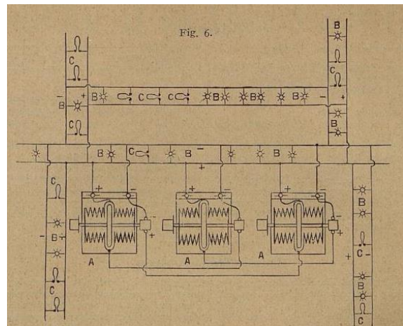
Rys. 5. Schemat równoległego połączenia lamp łukowych (B) i żarówek (C) z dynamo (A) w systemie Gülchera
