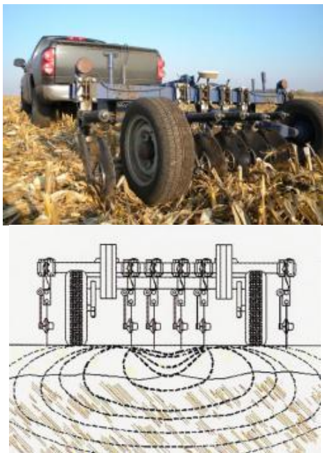
Fig. 2. EC Veris 3100 device
