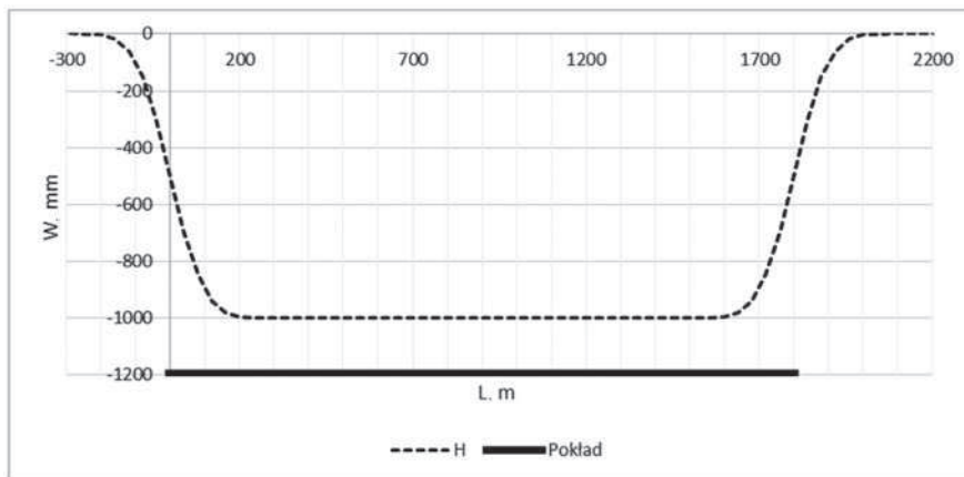
Rys. 7. Wyinterpolowana niecka obniżeniowa w przekroju poprzecznym A-A' (rysunek 5) przechodzącą przez środek abstrakcyjnej parceli
