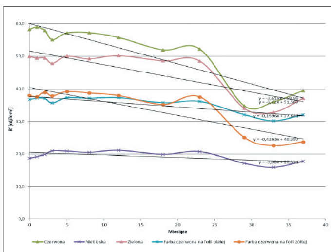
Rys. 3. Wyniki pomiarów współczynnika odbłasku folii typu 2, czerwonej, zielonej i niebieskiej (kąąt obserwacji 20°, kąąt oświetlenia \beta_v = +5^\circ ), podczas sztucznego starzenia
