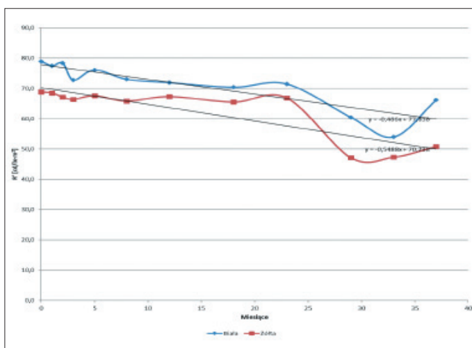
Rys. 2. Wyniki pomiarów współczynnika odbłasku folii typu 1, białej i żółtej (kąąt obserwacji 20°, kąąt oświetlenia \beta_v = +5^\circ ), podczas sztucznego starzenia
