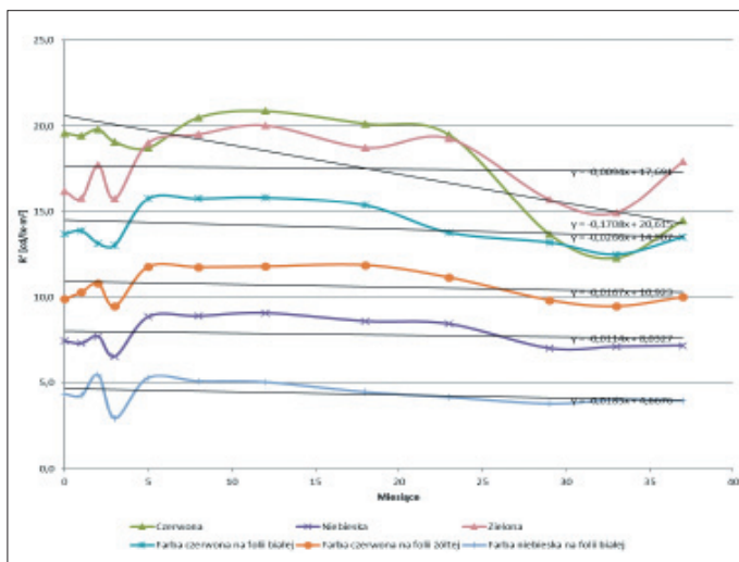
Rys. 1. Wyniki pomiarów współczynnika odbłasku folii typu 1, czerwonej, zielonej, niebieskiej (kąąt obserwacji 20°, kąąt oświetlenia \beta_v = +5^\circ ), podczas sztucznego starzenia
