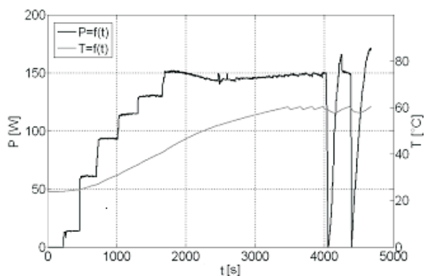
Rys. 6. Przebiegi generowanej mocy i wartości temperatury pracy stosu
