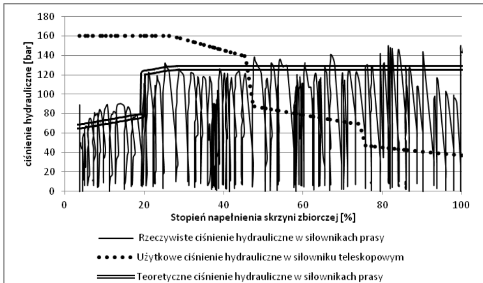
Rys. 7. Zestawienie wartości wielkości zmierzonych i teoretycznych dla procesu napełniania PUOP
