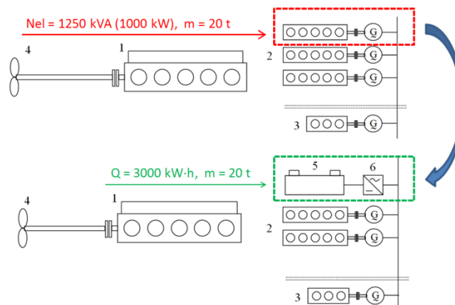
Rys.1. Koncepcja zamiany zespołu prądowórczego na baterię akumulatorów o podobnej masie 1 – silnik główny, 2 – zespoły prądowórcze, 3 – zespół awaryjny, 4 - śruba, 5 – bateria akumulatorów, 6 – falownik/prostownik
