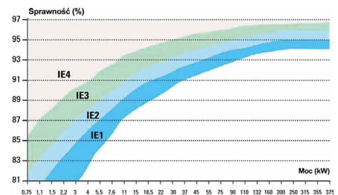
Rys. 2. Sprawność silników 4-biegunowych w poszczególnych klasach [6]
