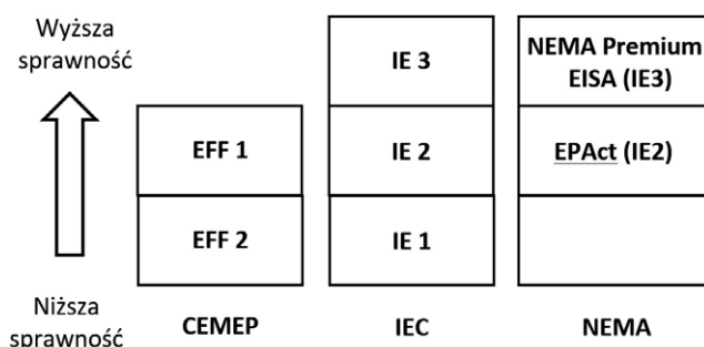
Rys. 3. Porównanie klas sprawności według (CEMEP ↔ IEC ↔ NEMA)
