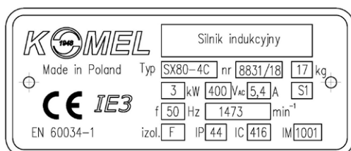
Rys. 4. Tabliczka znamionowa silnika Instytutu NiME Komel
