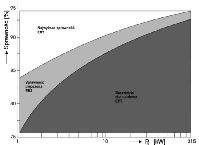
Rys. 1. Klasy sprawności silników o liczbie biegunów 2p = 4 według CEMEP
