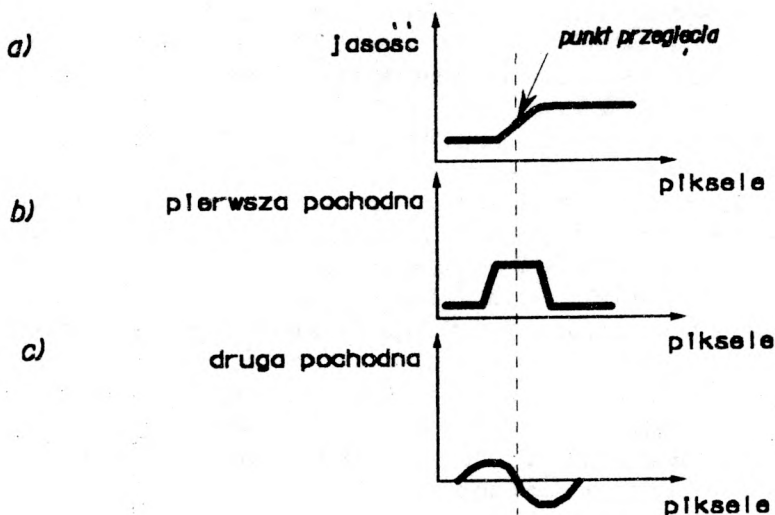
Rys.1: Krzywa przekroju mikrodensytometrycznego obrazu cyfrowego (a), oraz krzywe odpowiadające pierwszej (b) i drugiej pochodnej (c) krzywej przekrojowej. W miejscu, w którym oś przekroju przecina krzywą konturu rozgraniczającego na obrazie cyfrowym dwie powierzchnie o różnej jasności, występuje punkt przegięcia krzywej przekrojowej. W punkcie przegięcia wartość drugiej pochodnej funkcji zmienia znak, a zatem równa jest zero.
