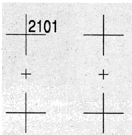
Rys.4: Fragment obrazu cyfrowego siatki reseau wykorzystywanej w badaniach testowych
