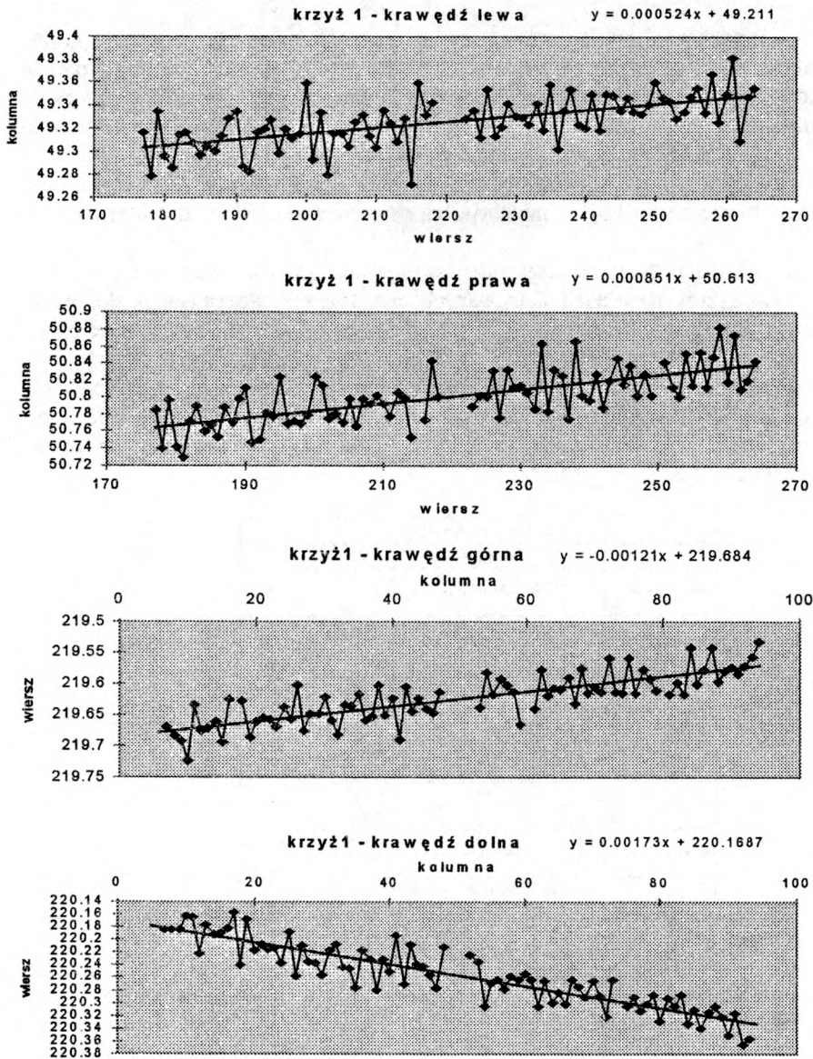
Rys.5. Zbiory punktów wyinterpolowanych z subpikselową dokładnością w przecięciu osi przekrojów mikrodensytometrycznych z krawędziami (liniami konturowymi) ramion obrazu przykładowego krzyża. Pokazano również linie proste aproksymujące punkty położone na krawędziach obrazów ramion krzyża. Ta aproksymacja jest drugim krokiem obliczeniowym zwiększającym pewność lokalizacji środka krzyża w układzie współrzędnych pikselowych.
