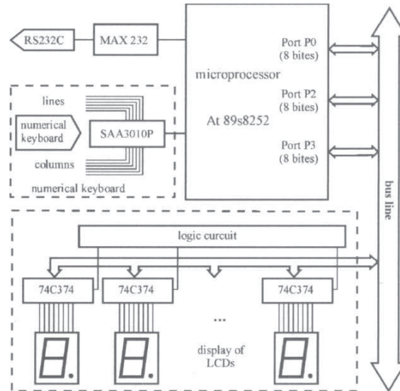
Fig. 2. Simplified electronic diagram of basic module Rys. 2. Uproszczony schemat elektroniczny modulu podstawowego
