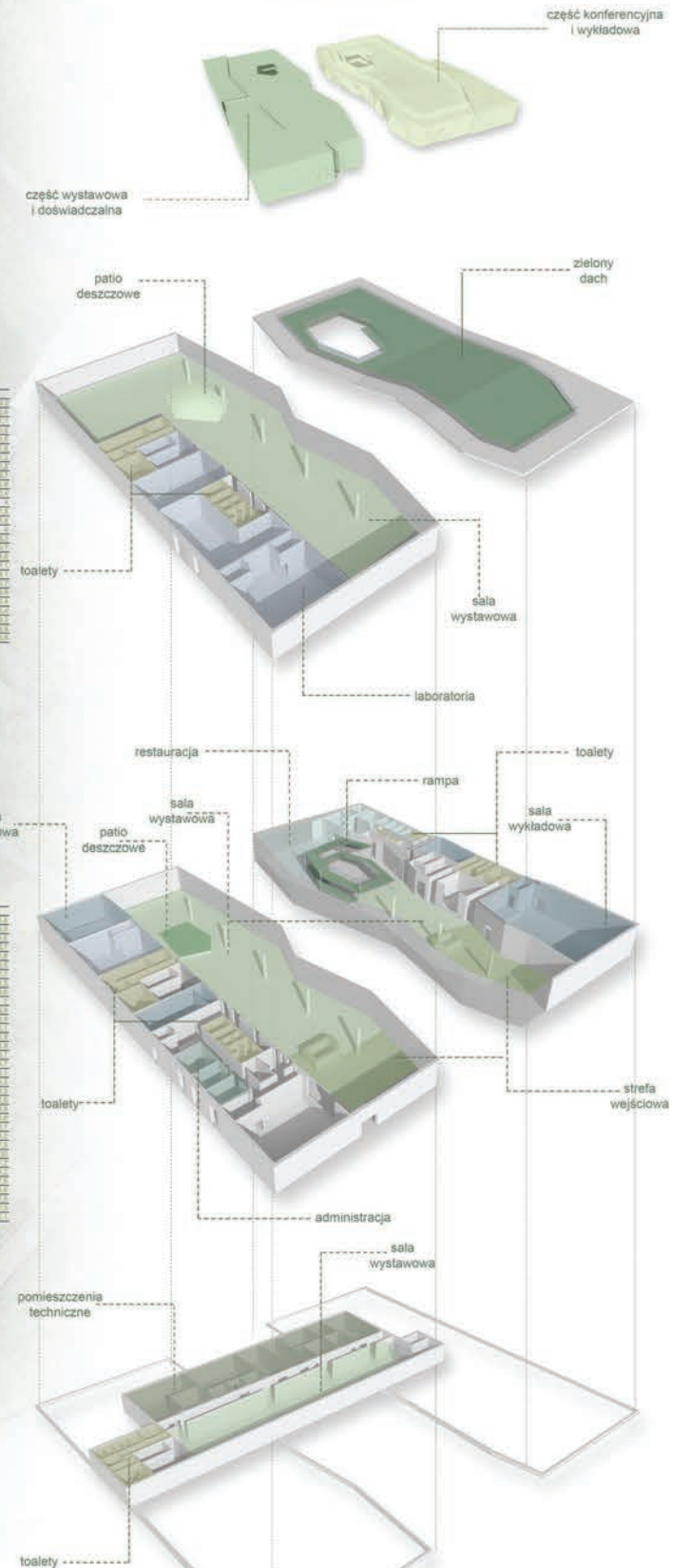
SCHEMAT FUNKCJONALNY Functional scheme
