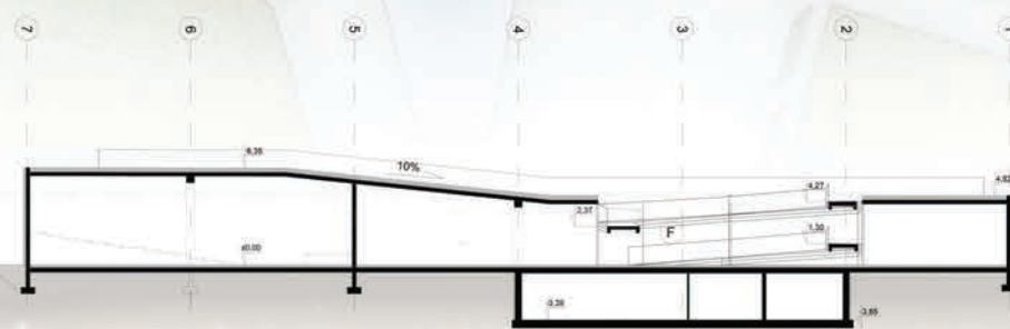
PRZEKRÓJ C-C 1:200 Section C-C 1:200
