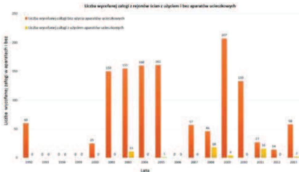
Rys. 7. Liczba wycofanej załogi z rejonów ścian, która użyla lub nie aparatów uciezkowych Fig. 7. Crew evacuated from the area of longwalls, who used and failed to use the rescue equipment
