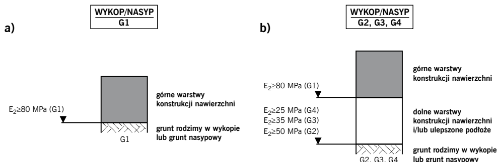
Rys. 2. Schemat układu warstw konstrukcji nawierzchni dla kategorii ruchu KR1-KR2 w wykopie i w nasypie oraz wymagane wartości wtórnych modułów odkształcenia na powierzchni warstw; a) w przypadku grupy nośności podłoża G1, b) w przypadku grupy nośności podłoża G2, G3 i G4
