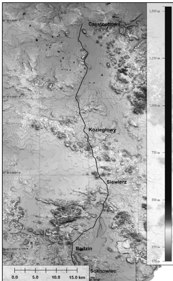
Ryc. 2. Numeryczny Model Terenu z zaznaczoną trasą S1 Sosnowiec-Częstochowa (67 km), (DTED 2, udostępniony przez WSK Warszawa 2005).
