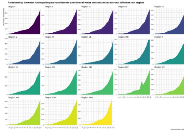
Fig 2. Relationship between hydrogeological coefficients and time of water concentration in the different rain regions of Vietnam [34] Rys. 2. Zależność współczynników hydrogeologicznych od czasu koncentracji wody w różnych regionach deszczowych Wietnamu [34]
