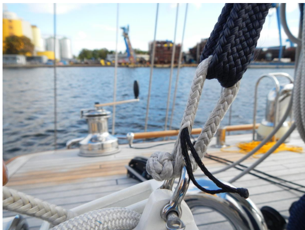
Rys. 6. Miękką szekla jako łącznik pomiędzy nokiem bomu a topenantą
