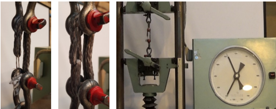
Rys. 14. Przebieg badań siły zrywającej na zawiesiu bezkońcowym typu U
