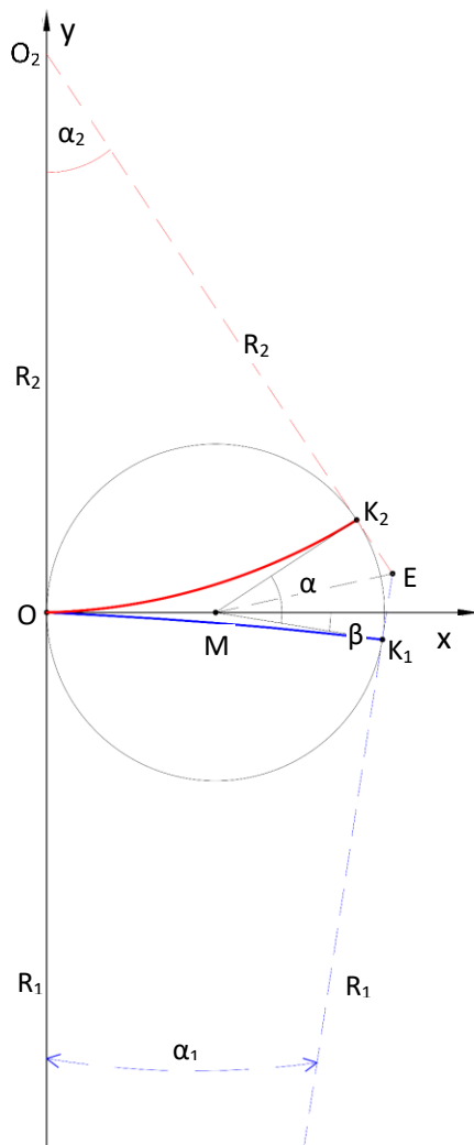
Rys. 4. Schemat łukowania rozjazdu zwyczajnego w wariacie II
