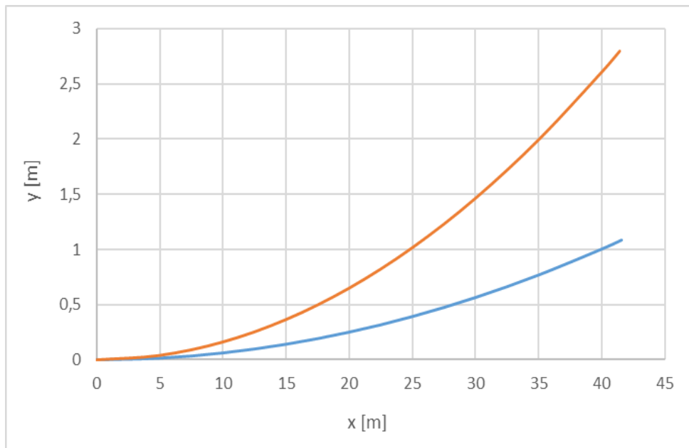
Rys. 3. Wykresy rzędnych poziomych toru zasadniczego i toru zwrotnego dla wariantu I łukowania rozjazdu 1 : 12 – 500 ( R_1 = 800 m, R_2 = 307,360 m) – w skali skażonej
