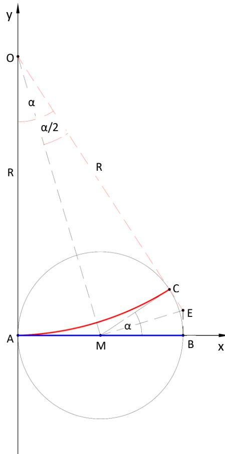
Rys. 1. Schemat rozjazdu zwyczajnego przed rozpoczęciem jego łukowania
