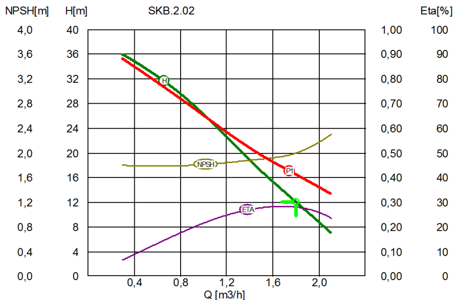
Rys. 8. Charakterystyki przepływowe wirowej pompy krążeniowej SKB 2.02 [11]
