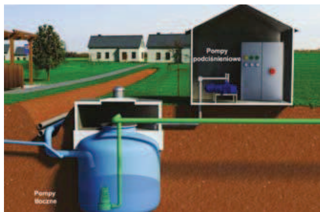
Rys. 4. Stacja podciśnieniowa [3]
