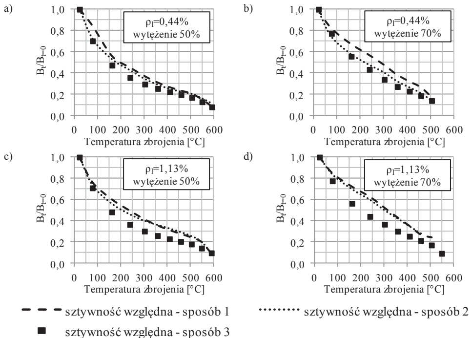
Rys. 7. Wykresy względnego obniżenia sztywności przekroju z ogrzewanym zbrojeniem: a) \rho_f=0,44\% , wyteż. 50%, b) \rho_f=0,44\% , wyteż. 70%, c) \rho_f=1,13\% , wyteż. 50%, d) \rho_f=1,13\% , wyteż. 70%;
