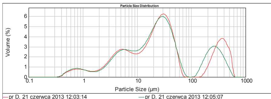
Rys. 4. Wielkości cząstek dla próbki D: d_1 = 0,79 \mu\text{m} , d_2 = 5,6 \mu\text{m} , d_3 = 31,7 \mu\text{m} , d_4 = 355 \mu\text{m}
