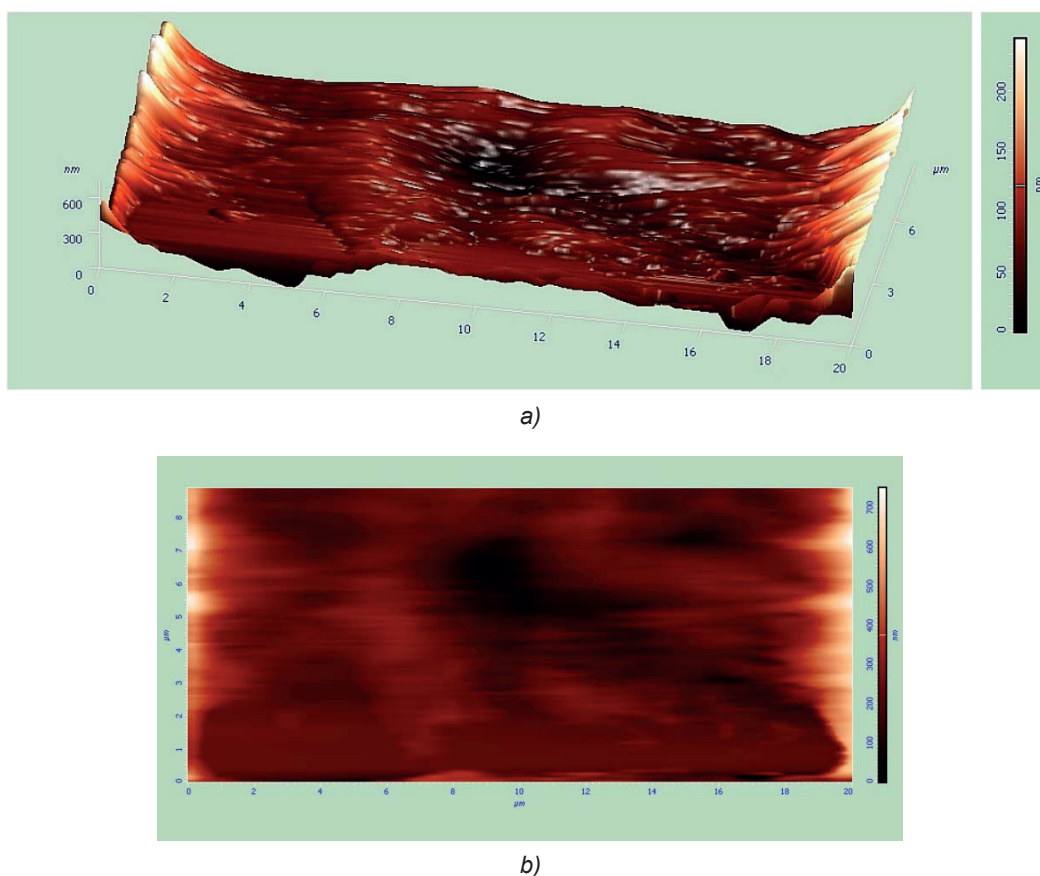
Rys. 5. Topografia powierzchni wosku: a) trójwymiarowy wykres nierówności b) mapa topografii powierzchni Fig. 5. Wax surface topography: a) 3D graph of surface irregularities b) surface topography map
