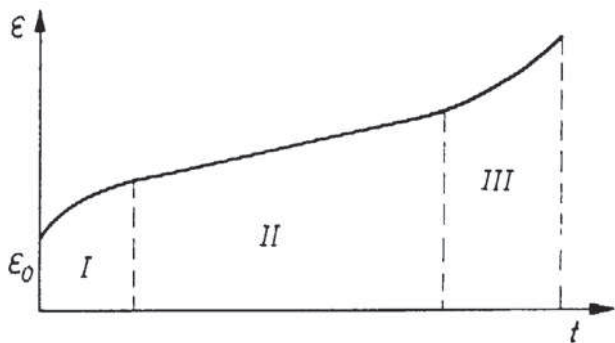
Rys. 6. Typowa krzywa wzdłużnego odkształcania się liny I, II, III - nieustalony, ustalony i przyspieszony okres odkształcania
