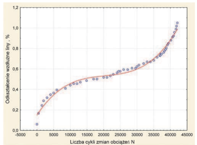
Rys. 9. Wykres narastania wzdłużnych odkształceń liny trójkątnośliskowej \varnothing 50 mm podczas badania zmęczeniowego Fig. 9. Graph of mounting longitudinal strains of the triangular-strand rope \varnothing 50 mm during a fatigue test
