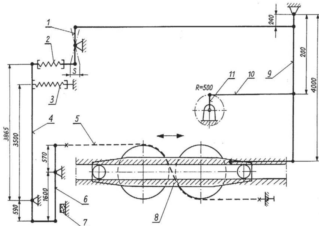
Rys. 1. Schemat kinematyczny maszyny zmęczeniowej P4-GIG-2
