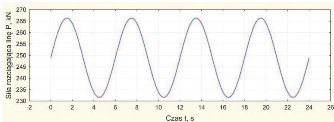
Rys 4. Przebieg obciążeń rozciągających cyklicznie zmiennych liny trójkątnospłotkowej \varnothing 50 mm w badaniach zmęczeniowych
