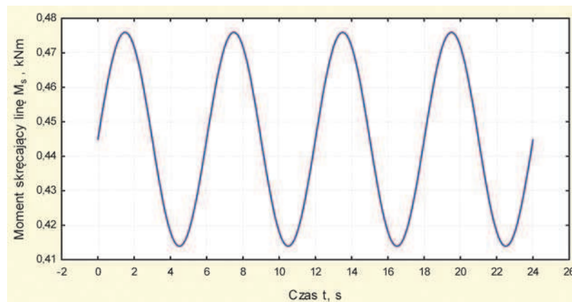
Rys. 5. Przebieg cyklicznie zmiennego momentu skręcającego liny dwuwarstwowej \varnothing 46 mm w badaniach zmęczeniowych
