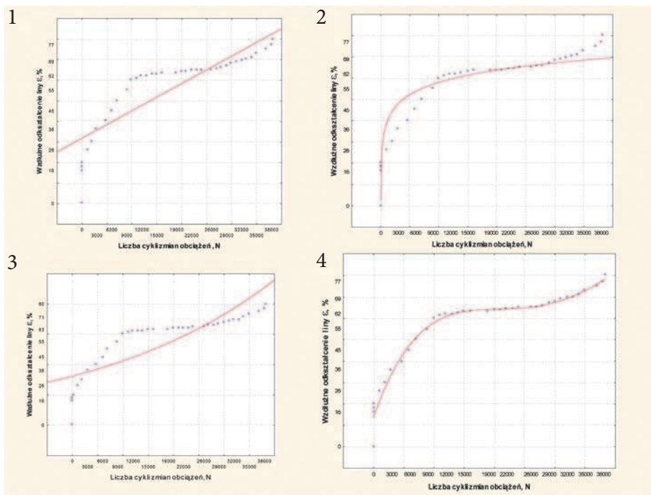
Rys. 7. Punkty odwzorowujące wyniki pomiarów oraz krzywe empiryczne (regresyjne) \epsilon = f(N) narastania wzdłużnych odkształceń liny \varnothing 46\text{mm} badanej w warunkach złożonych obciążeń cyklicznie zmiennych
