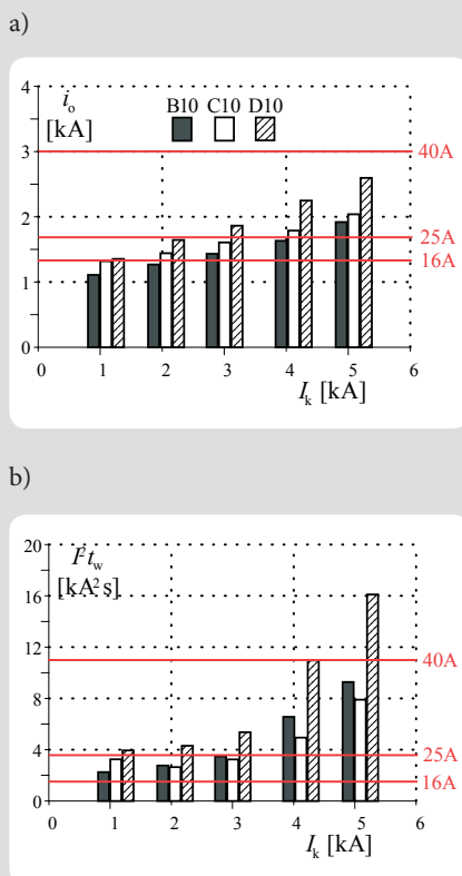
Rys. 6. Prądy ograniczone i_0 (a) i całki Joule'a wyłączenia \int I^2 dt (b) wyłączników o charakterystykach B, C, D i prądzie znamionowym I_n = 10 A oraz największy dopuszczalny prąd szczytowy i całka Joule'a dla wyłączników różnicowoprądowych o I_n = 16, 25 i 40 A
