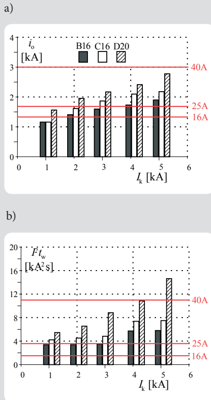
Rys. 5. Prądy ograniczone i_0 (a) i całki Joule'a wyłączenia \int I^2 dt (b) wyłączników B16, C16, D20 oraz największy dopuszczalny prąd szczytowy i całka Joule'a dla wyłączników różnicowoprądowych o I_n = 16, 25 i 40 A
