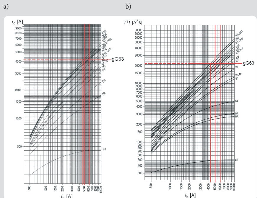
Rys. 8. Prąd ograniczony i_0 (a) i całka Joule'a wyłączenia \int I^2 dt (b) wyłączników nadprądowych instalacyjnych typu B [6]
