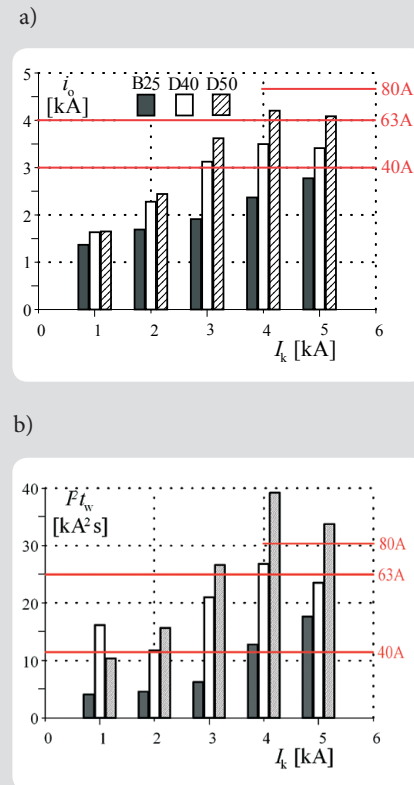
Rys. 7. Prądy ograniczone i_0 (a) i całki Joule'a wyłączenia \int I^2 dt (b) wyłączników B25, D40, D50 oraz największy dopuszczalny prąd szczytowy i całka Joule'a dla wyłączników różnicowoprądowych o I_n = 40, 63 i 80 A
