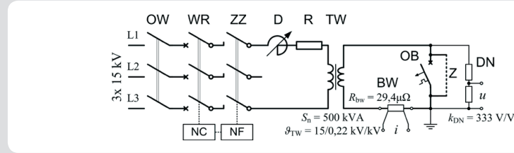
Rys. 2. Schemat stanowiska do badań wyłączników nadprądowych instalacyjnych
