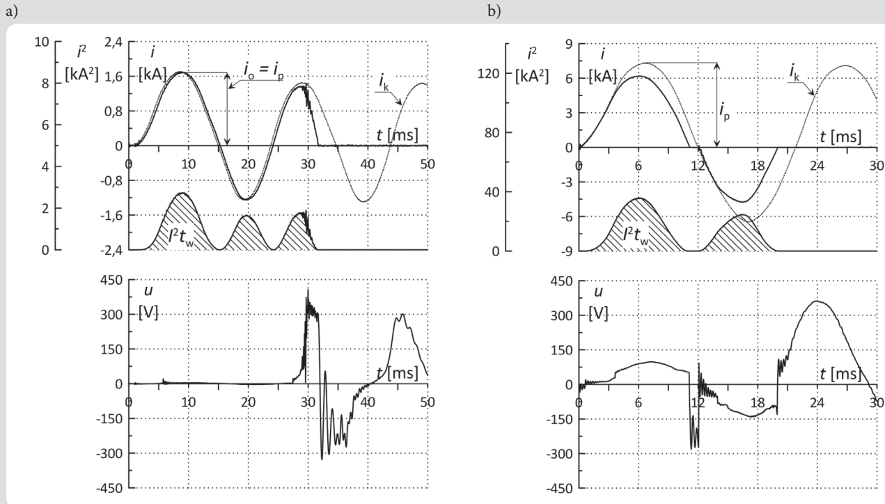
Rys. 4. Wyłączanie prądu zwarciego przez wyłącznik nadprądowy instalacyjny; a) wyłącznik D40, I_k = 1,0 kA, i_p = 1,7 kA, i_o = 1,7 kA, I^2t_w = 31,3 kA 2 s b) wyłącznik C100, I_k = 4,8 kA, i_p = 7,1 kA, i_o = 6,0 kA, I^2t_w = 144,6 kA 2 s; brak ograniczania prądu zwarciego
