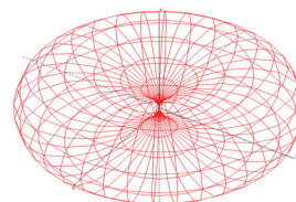
Rys. 1. Charakterystyka promieniowania dipola półfalowego (Xnecview)
